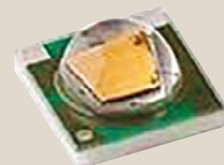
Afmetingen 1 LED: 3.45 x 3.45 x 2.00 mm
